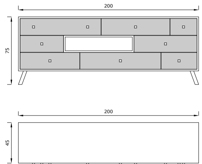
szafka RTV
